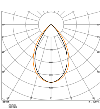
LB FLEX 1500 P 73W 840 N
