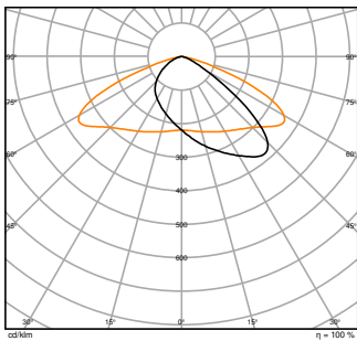
FL PFM DA 50W 3000K ASYM 45X140 BK
