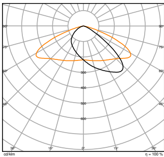
FL PFM DA 200W 4000K ASYM 45X140 BK
