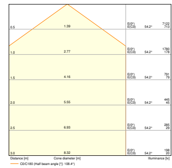
BATTEN CBO 1200 V 36W MS 840 WT
