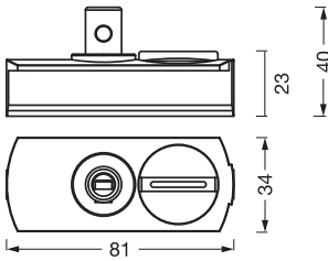
TRACKLIGHT PENDANT CONNECTOR
